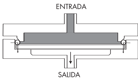
Mecanismo de sellado
