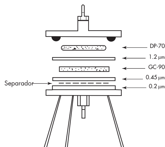
Una típica pila de serie que incorpora prefiltros, membranas y separadores de malla de poliéster.
